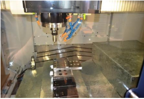
精密機械技術科はチタンのプレートに、マシニングセンタでイニシャルを加工
